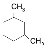
1,3-dimetilciclohexano
