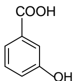
ácido m -hidroxibenzoico
