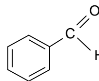
Benzaldehído
