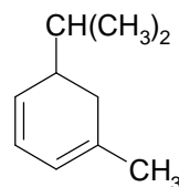
1-metil-5-isopropil-1,3-ciclohexadieno
