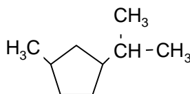
3-isopropil-1-metil-ciclopentano
