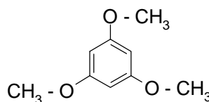
1,3,5 -trimetoxibenceno
