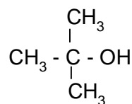
Alcohol terbutílico
