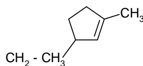
3-etil-1-metil-1-ciclopenteno
