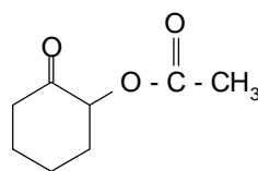
2-acetoxi-ciclohexanona
