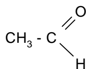
Etanal Acetaldehído
