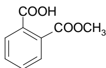
Ácido o-carbometoxibenzoico
